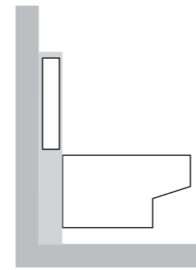
Конзолно решение, предсидна монтажа или монтажа во сид
