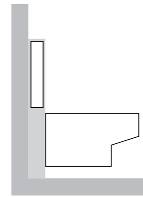
Конзолно решение, предсидна монтажа
